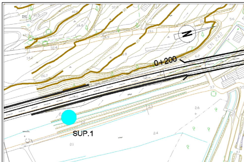
Figura 17 – Ponto de monitorização SUP1, localizado no Colector Periférico (km 0+100)
